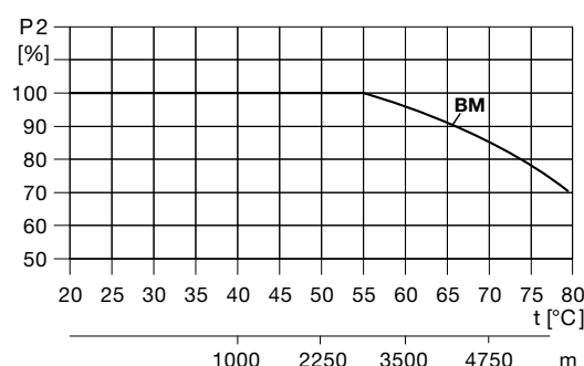
Abb./Fig./Afb. 1 Zusammenhang zwischen der Motor- ausgangsleistung ( P_2 ) und der Umgebungstemperatur-Aufstellungshöhe.
